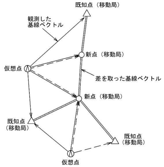
重複辺による点検をする場合
