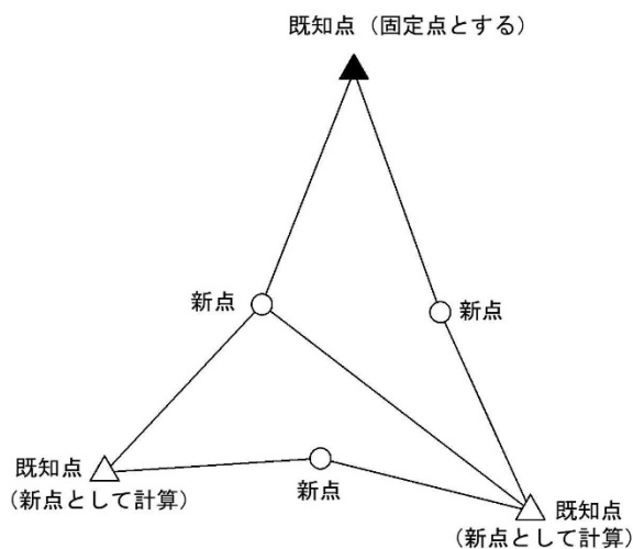
仮定三次元網平均
