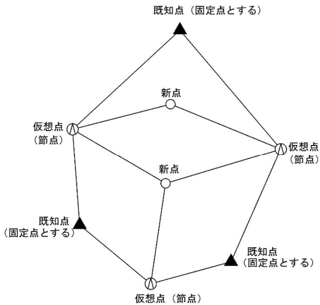
三次元網平均（直接観測法）
