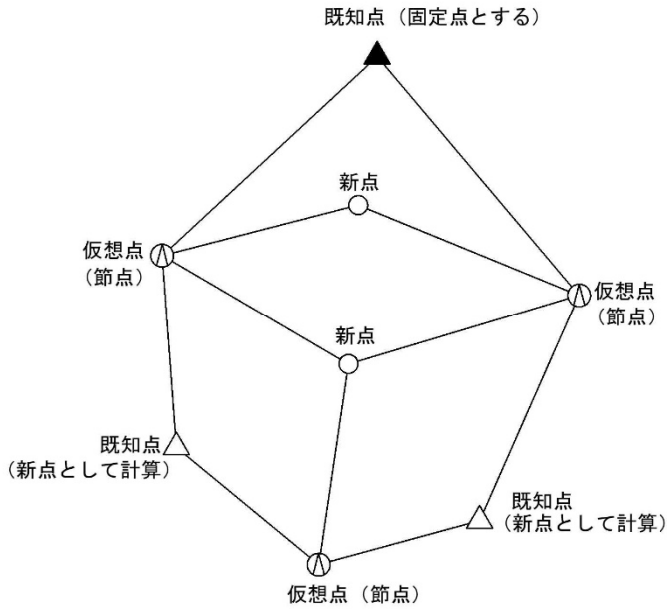
仮定三次元網平均（直接観測法）
