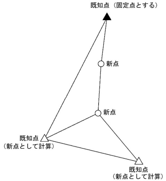
仮定三次元網平均（間接観測法）
